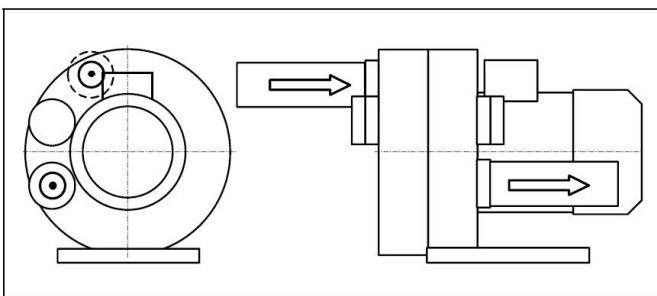
Рис. 3: Двухступенчатые вакуумные насосы/компрессоры с двумя рабочими колесами
