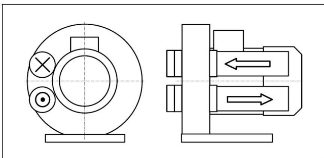
Рис. 2: Вакуумные насосы/компрессоры с одним рабочим колесом
