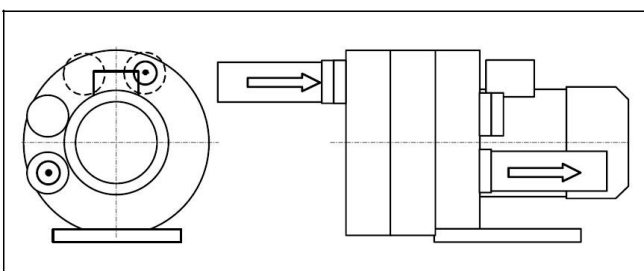
Рис. 4: Трехступенчатые вакуумные насосы/компрессоры с тремя рабочими колесами
