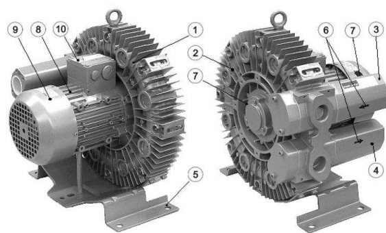
Рис. 1: Конструкция вихревой воздуховулки (вакуумного насоса/компрессора)
